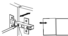
調整ねじ
