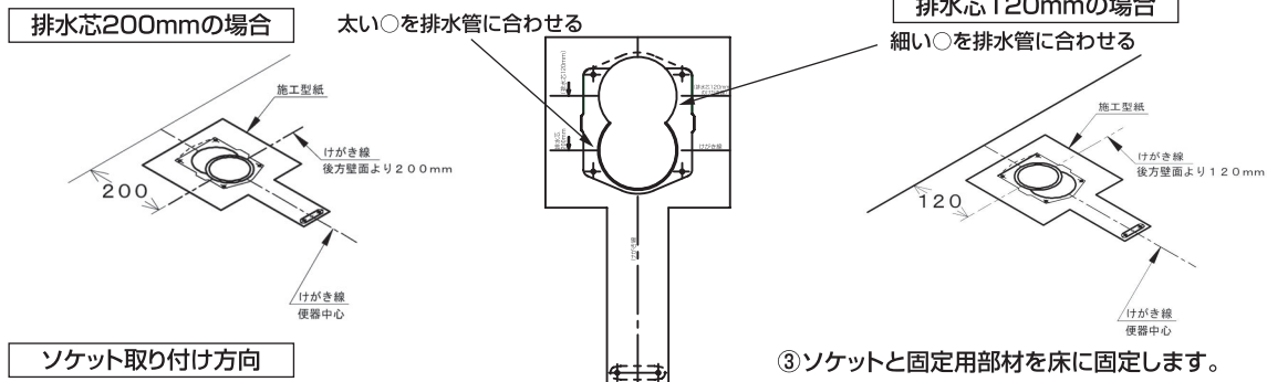
排水芯200の場合
