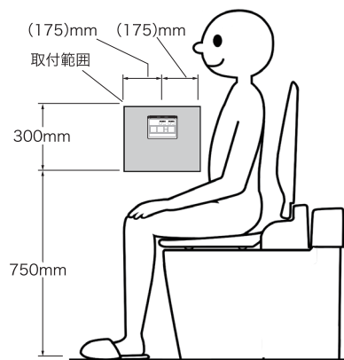
(リモコン取り付け参考図)
