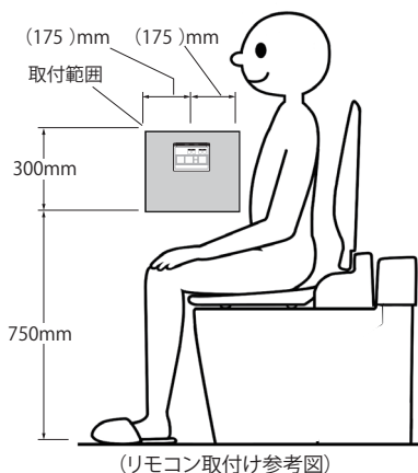
(リモコン取付け参考図)
