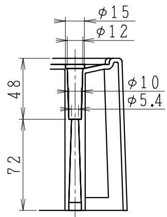
ねじ部詳細図 (S = 1 : 3)
