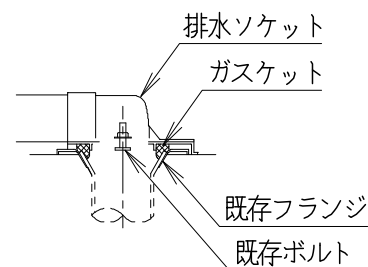
排水ソケットとフランジ部の固定
