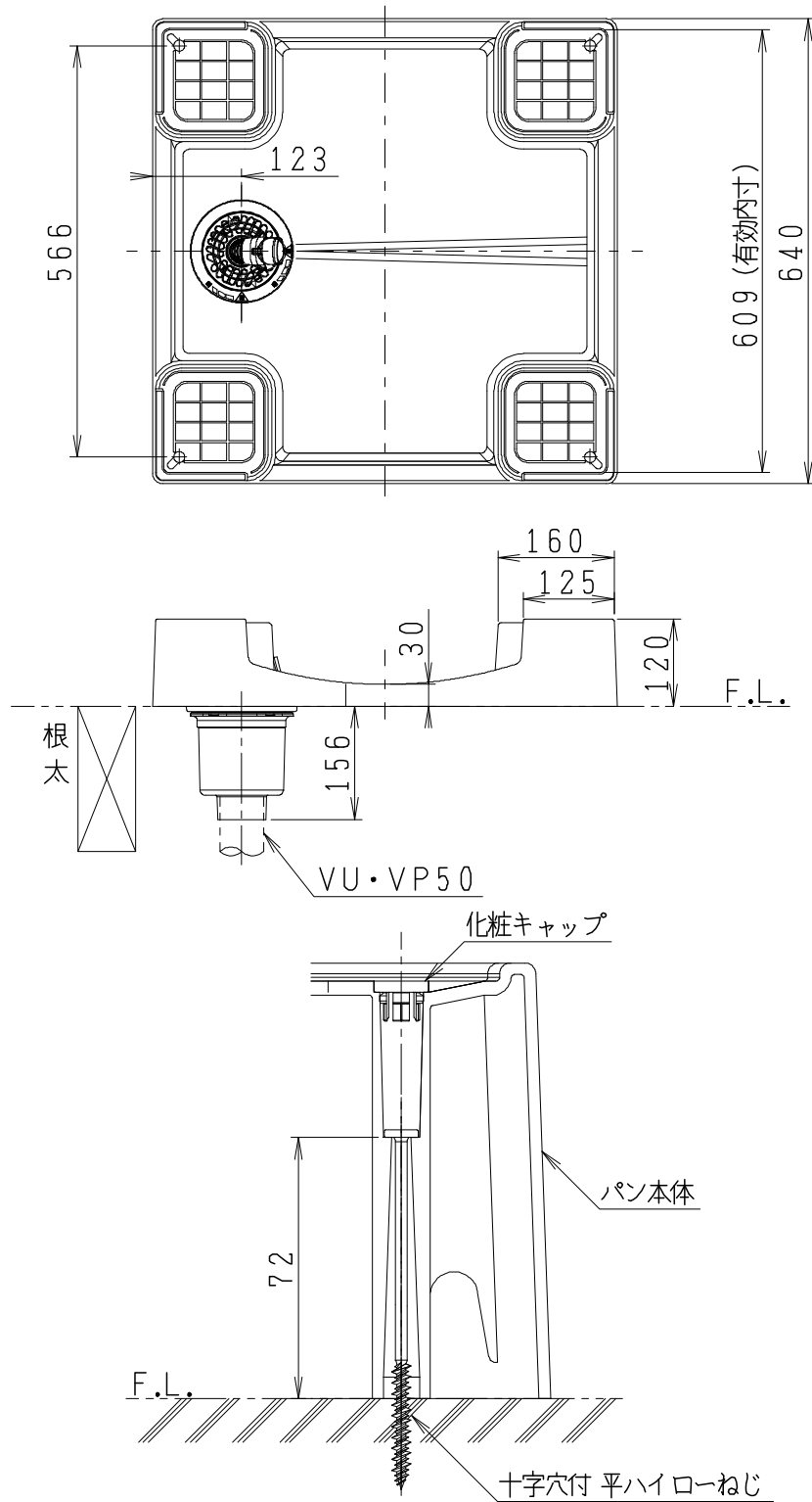
防水パン固定部詳細図 (S = 1 : 2)
