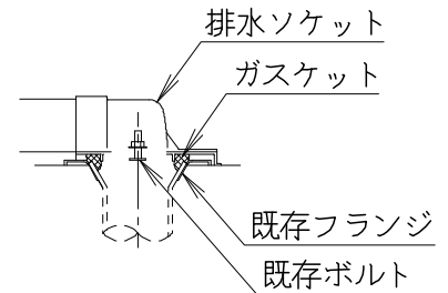
排水ソケットとフランジ部の固定
