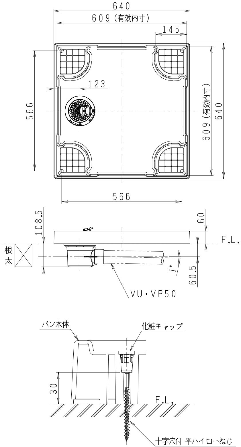
防水パン固定部詳細図
