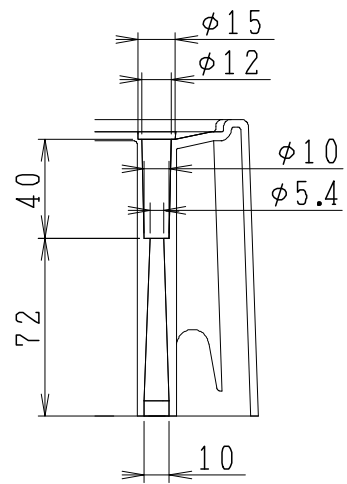
ねじ部詳細図 (S = 1 : 3)
