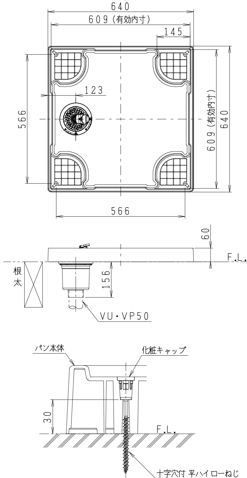
防水パン固定部詳細図
