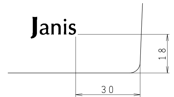
A部詳細図 S:1/1 転写マーク貼付位置
