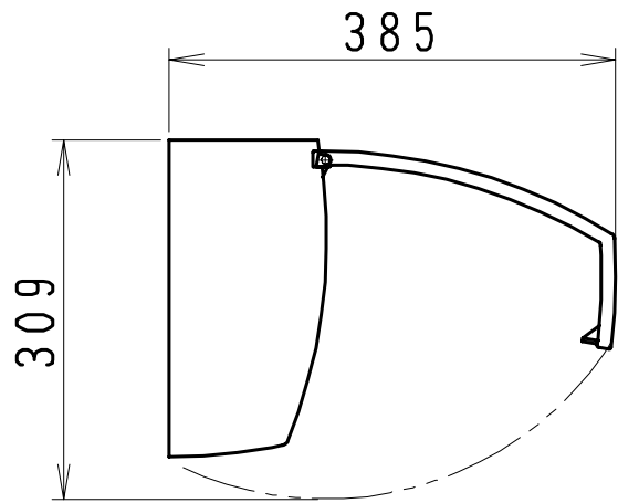
扉開閉図
