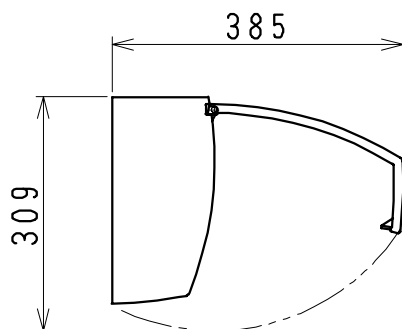
扉開閉図
