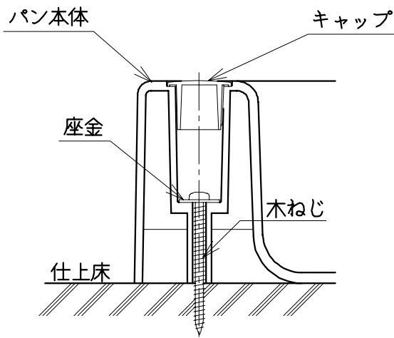
防水パン固定部詳細図
