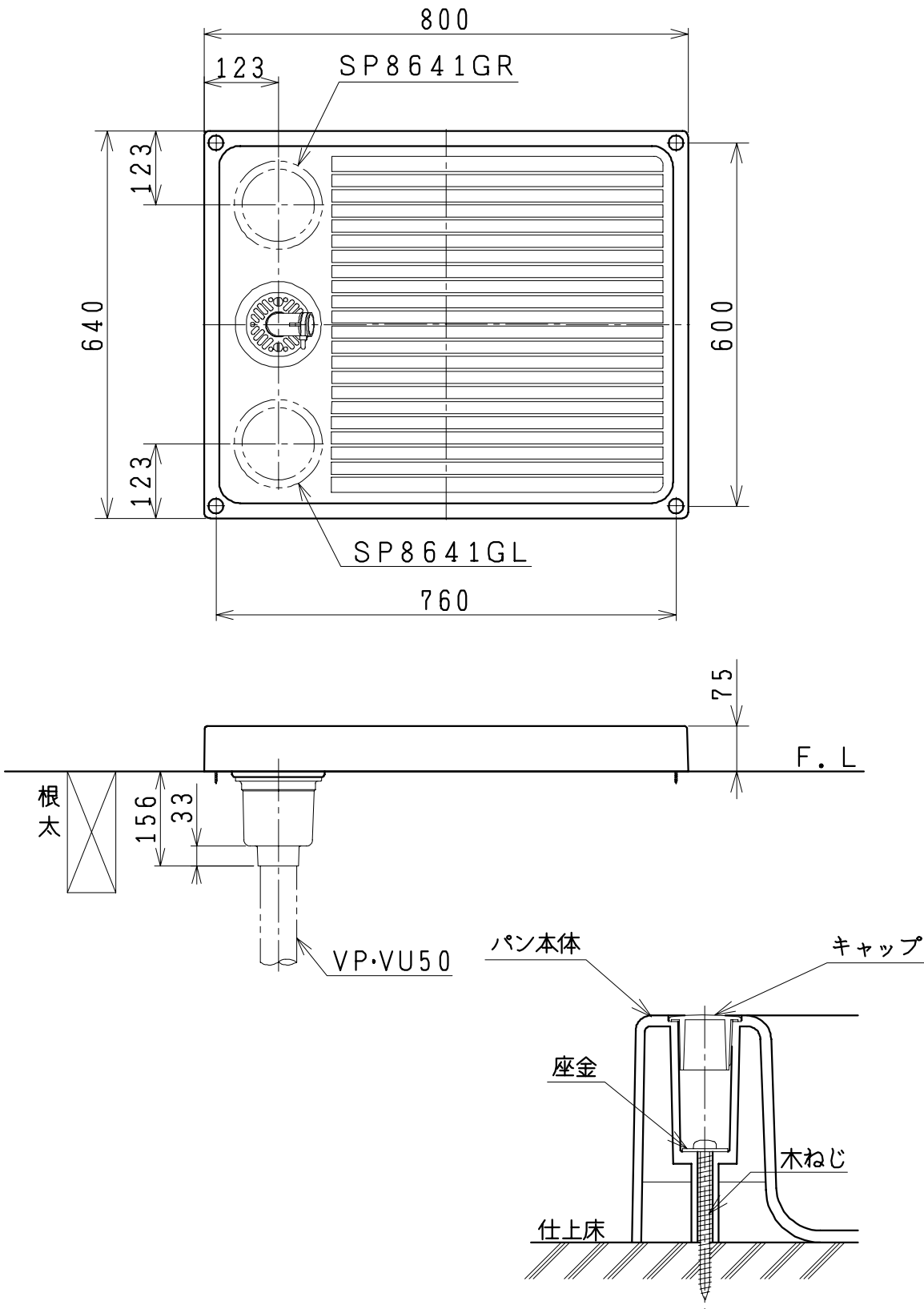
防水パン固定部詳細図
