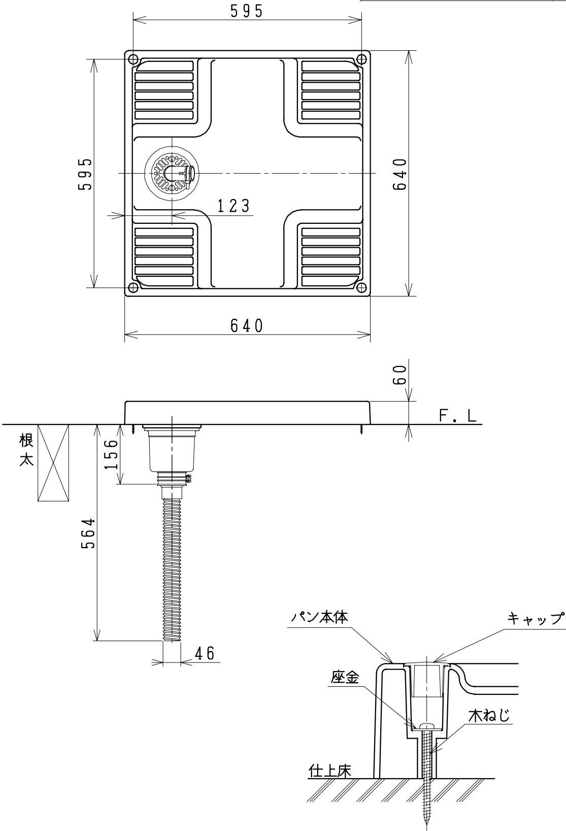
防水パン固定部詳細図
