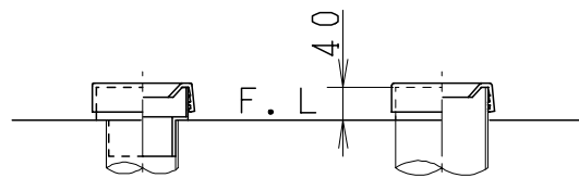
VU、VP75の場合 床面カット
