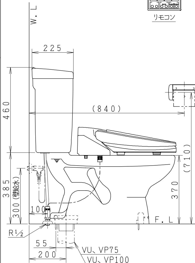
VU、VP75の場合 床面カット
