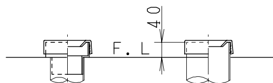
VU、VP75の場合 床面カット
